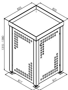
Außenmaß 1 x 240 Liter, Wanne
