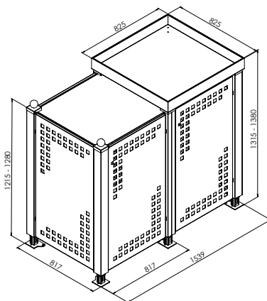
Außenmaß 2 x 240 Liter, Wanne
