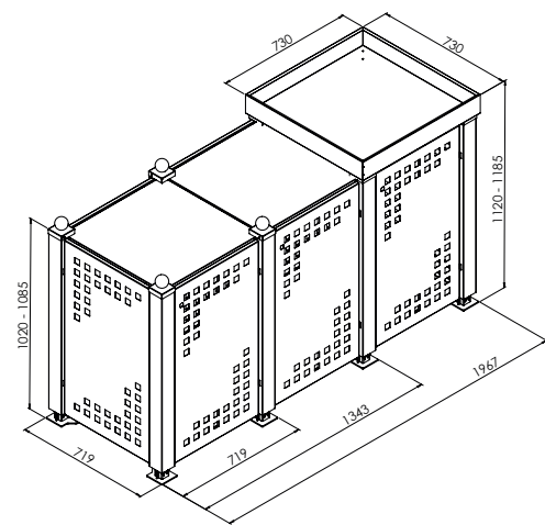
Außenmaß 3 x 120 Liter, Wanne
