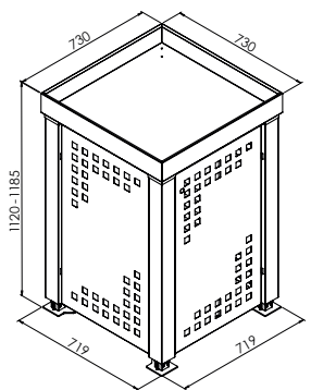
Außenmaß 1 x 120 Liter, Wanne
