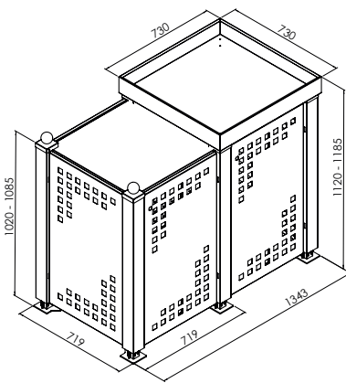
Außenmaß 2 x 120 Liter, Wanne
